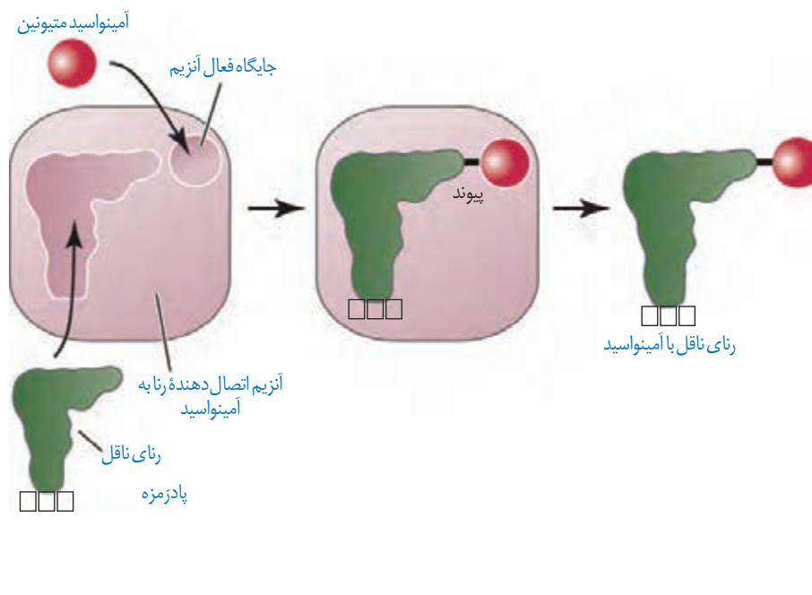
شکل ۹- نحوه پیوستن آمینواسید به رنای ناقل مربوط به خود توسط آنزیم ویژه آن
