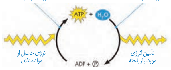
شکل ۲- تبدیل ADP و ATP به یکدیگر
